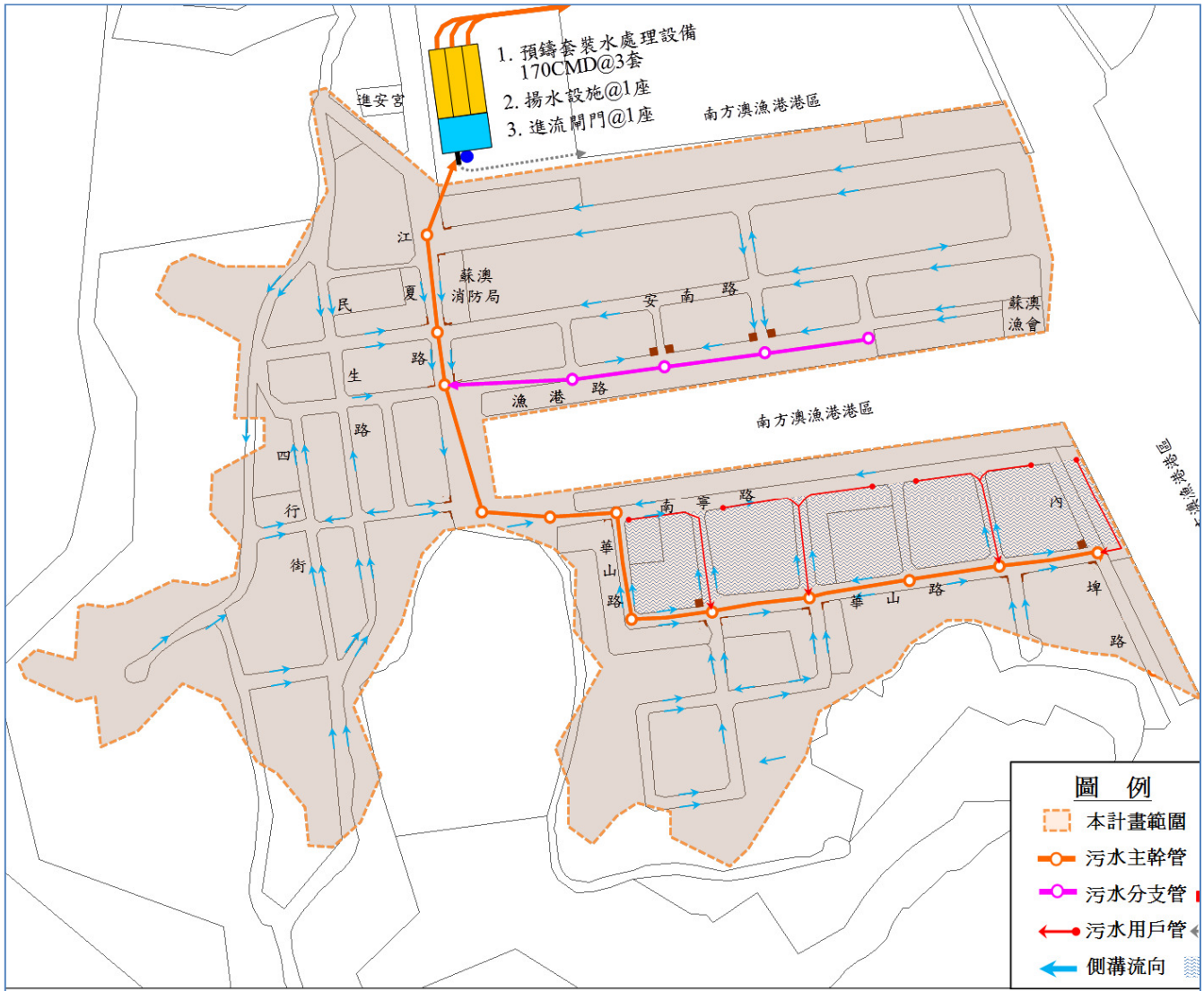
蘇澳鎮南方澳漁港區域水體環境水質改善整體計畫 (南方澳漁港區周邊污水截流工程管線施工路線圖)
