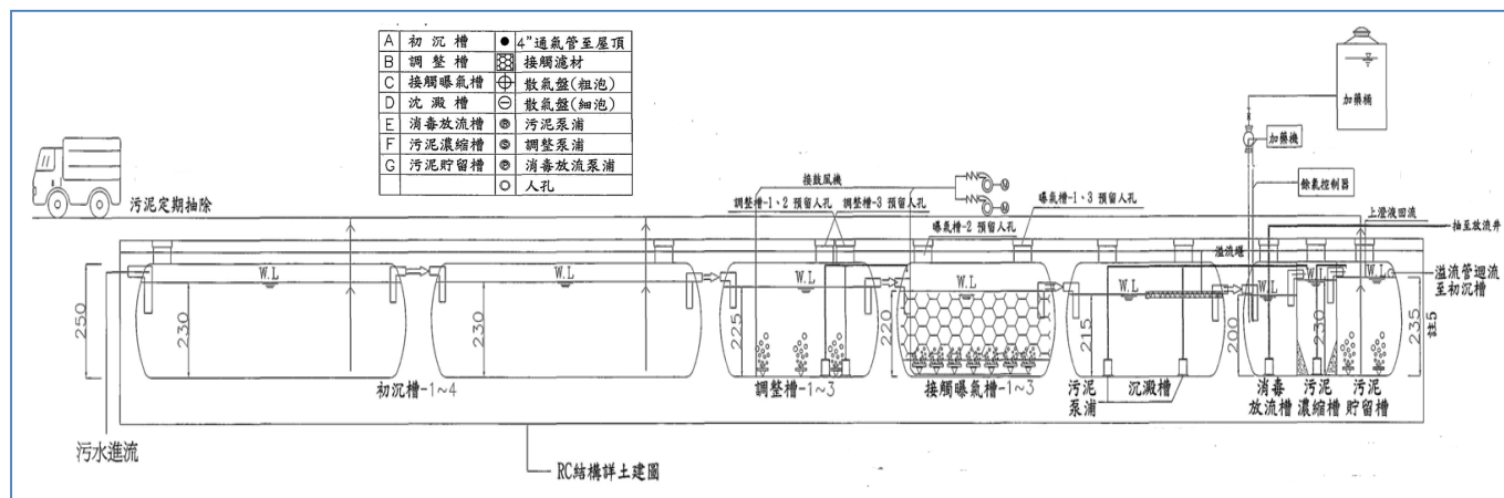
南方澳魚港區聚落污水處理設施工程污水處理流程剖面圖
