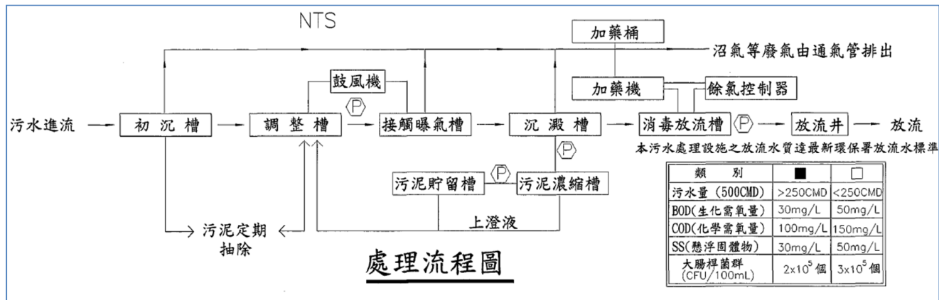
南方澳魚港區聚落污水處理設施工程污水處理流程圖
