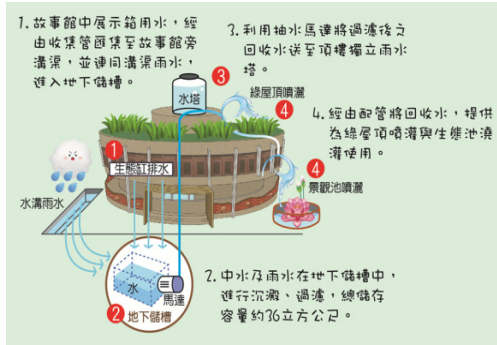
中水回收系統
